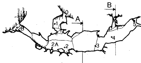
SEZIONE LONGITUDINALE
